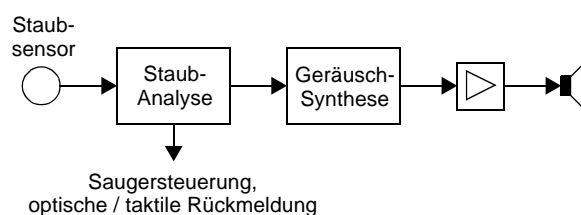
Abb. 1 Aufbau des Systems zur Aktiven Geräuschgestaltung bei Staubsaugern basierend auf einer Messung des Staubflusses
