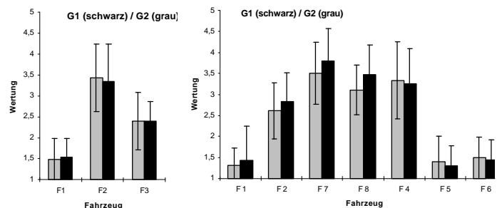
Abb. 2 Ergebnisse Phase 2 und 3: Beurteilungen der Ausgeprägtheit des Getrieberasseln aus Feld (links) und Labor (rechts). Helle Balken: Gruppe, die zuerst im Feld war; dunkle Balken: Gruppe, die zuerst im Labor war.
